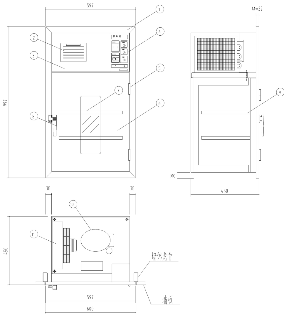
图示面框和墙面齐平
